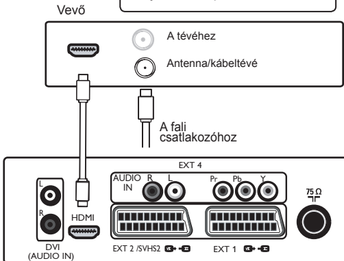
A TV alsó részén található csatlakozók
