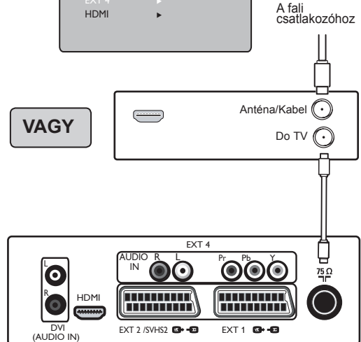
A TV alsó részén található csatlakozók
